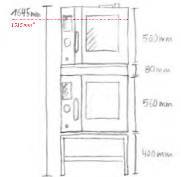
KombiMix-Station mit JOKER, Bedienung seitlich auf Untergestell 400mm.
